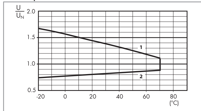
R 46 - Campo de funcionamiento de la bobina (AC) en función de la temperatura ambiente
